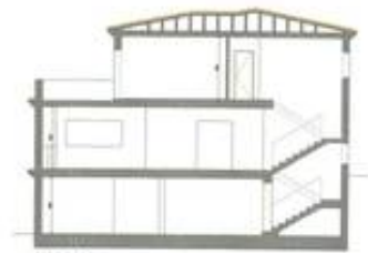
SECCION 1-1
