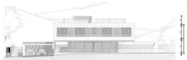
ALZADO SURESTE
