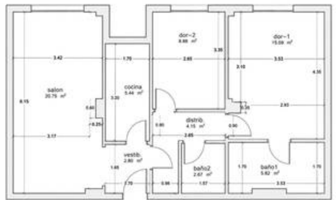
PLANTA VIVIENDA : 1/50 ESTADO REFORMADO
